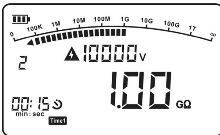
图 5：测试状态液晶显示界面
