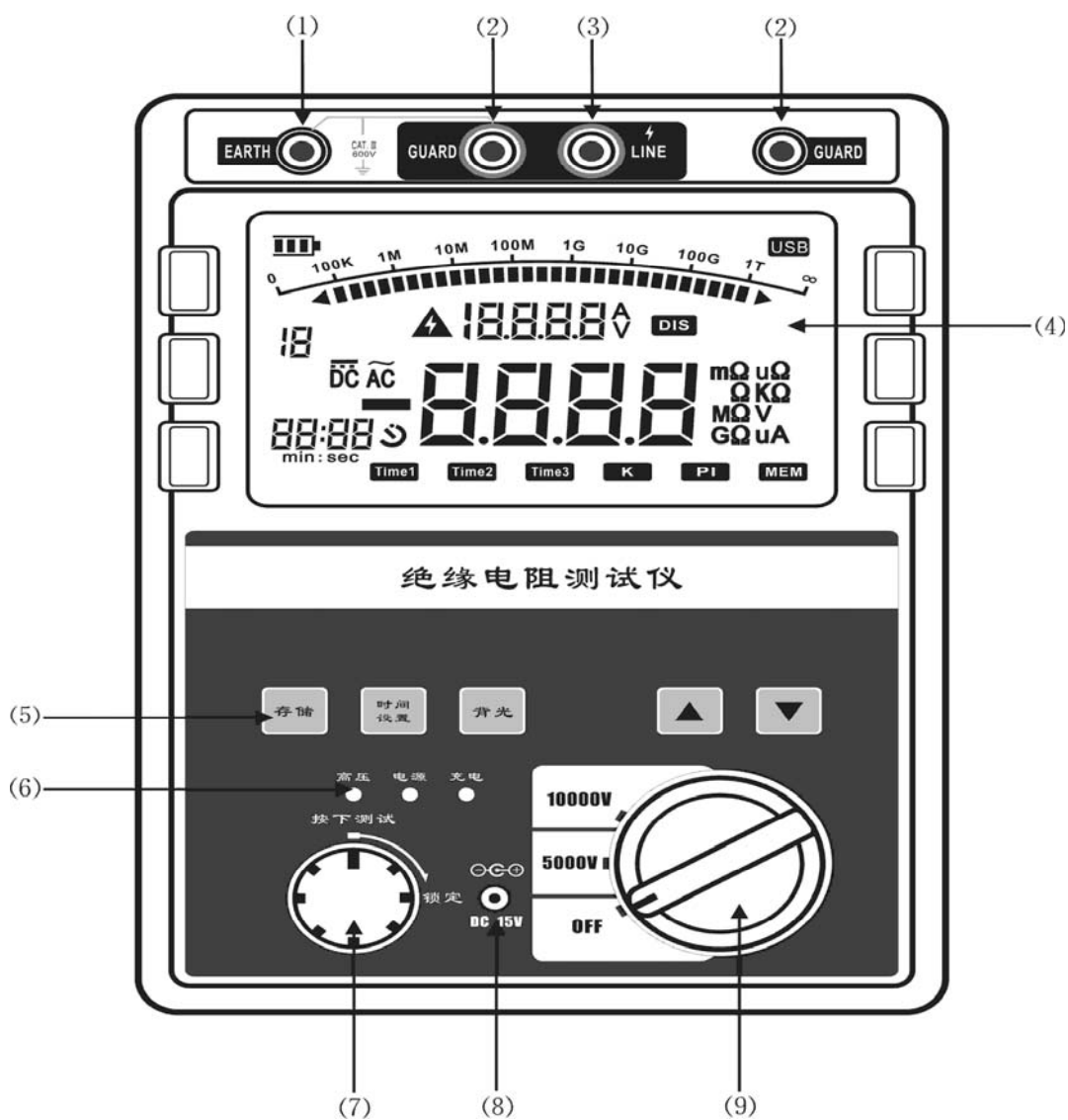
图 1: ZQBC-IV 系列面板结构说明
